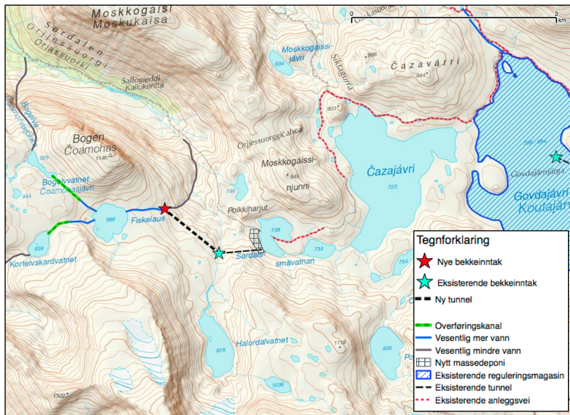
Figur 3.3. Kart som viser kanaler, tunnel og bekkeinntak i Poikkiharjutoverføringen samt eksisterende anlegg.
